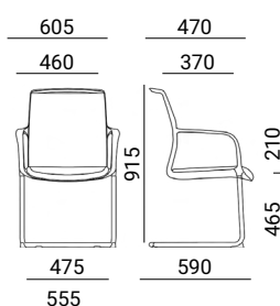
Join slede
